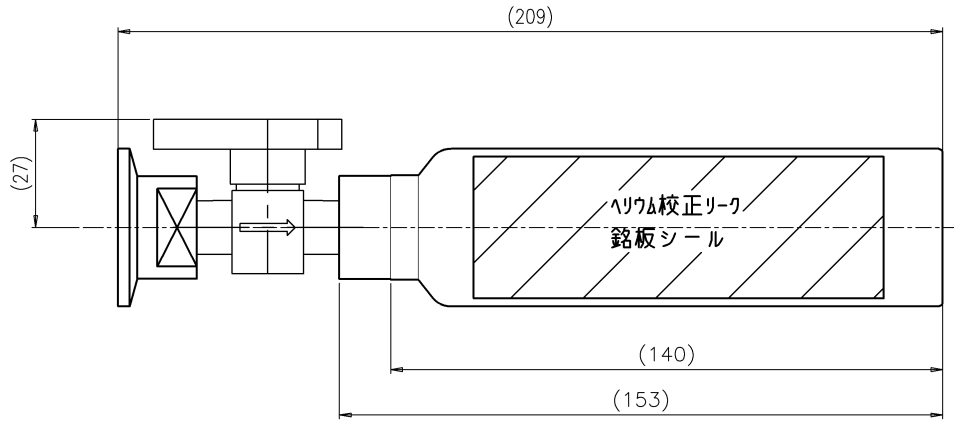
新校正リーク：ASL-25V 外観図
