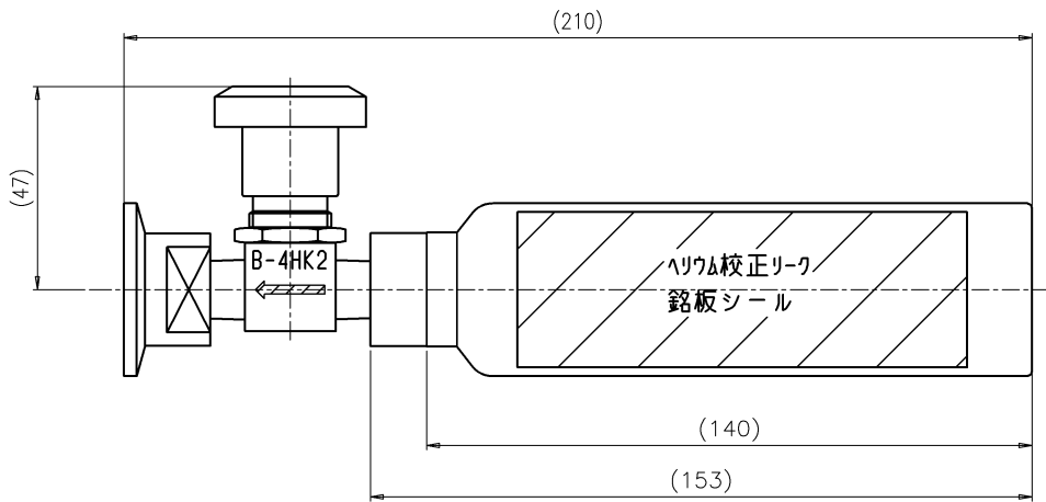
旧校正リーク：ASL-25V 外観図
